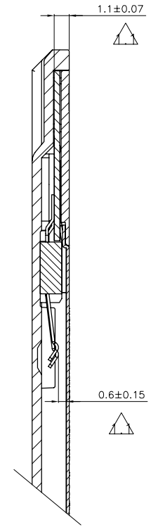
SECTION A-A SCALE 2:1
