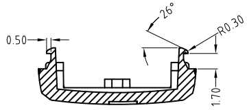
截面B-B
